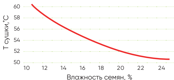
Температура сушки семян в зависимости от уборочной влажности рапса
