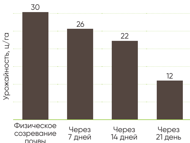
Влияние сроков сева на урожайность ярового рапса
